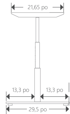
Piétement à 2LV-29 [UPMOD-2LV-29] vue latérale
