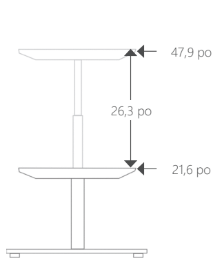
Piétement à 2LV [UPMOD-2LV-22 & UPMOD-2LV-29] Plage de réglages de hauteur
