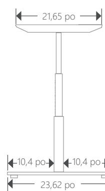
Piétement ES [UP-ES] vue latérale
