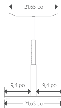
Piétement à 2LV-22 [UPMOD-2LV-22] vue latérale
