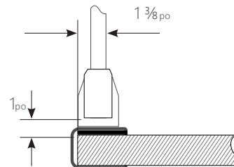
Support de fixation par pinces [CM]
