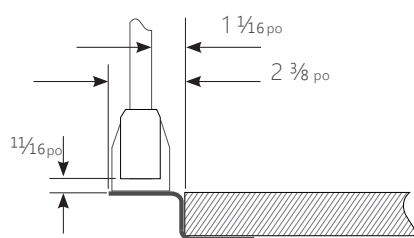
Support avec piètement autoportant [FL]
