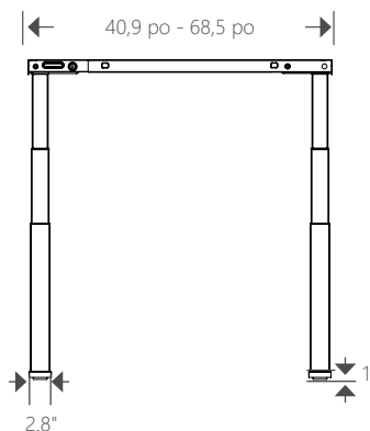
Piétement ES [UP-ES] vue avant
