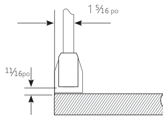
Coque de fixation à montage direct [DM]
