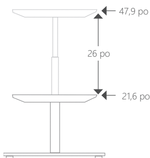
Piétement ES [UP-ES] Plage de réglages de hauteur
