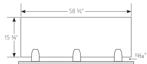
ex. PRIVACY-UNF-01-16X60 illustré avec 3 supports de montage direct en surface
