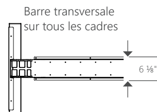
Piétement ES [UP-ES] vue latérale
