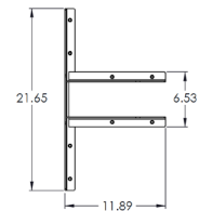
Piétement à 2LV-29 [UPMOD-2LV-29] vue latérale
